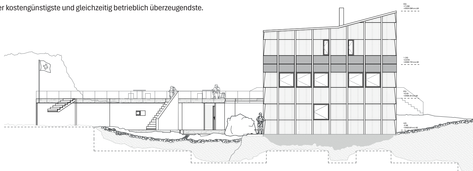
Ansicht Süd-Ost
